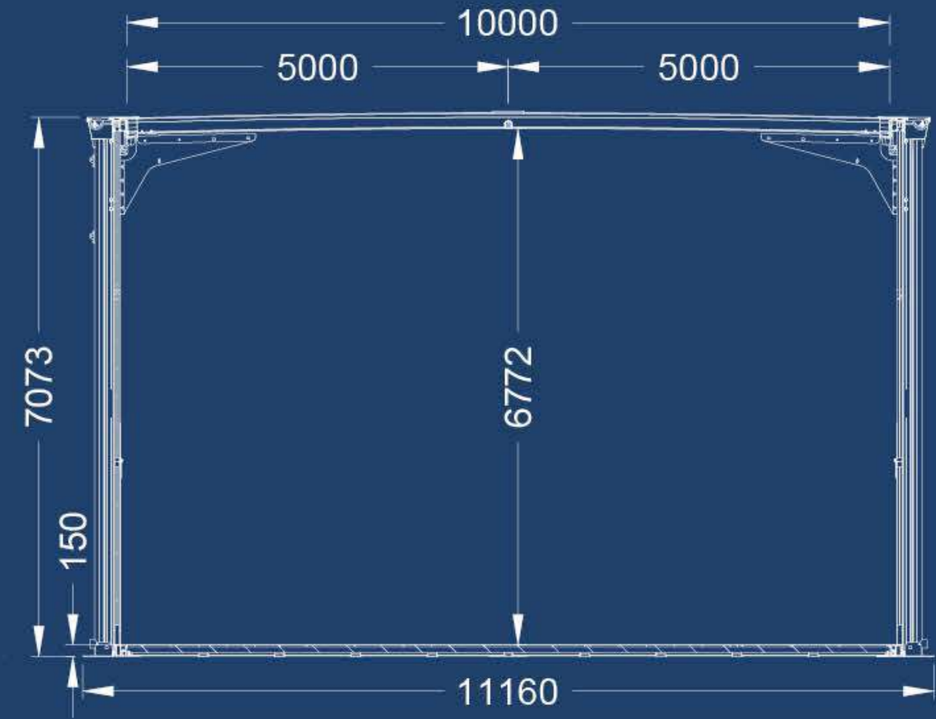
Pórtico de 10m sin mezzanina
