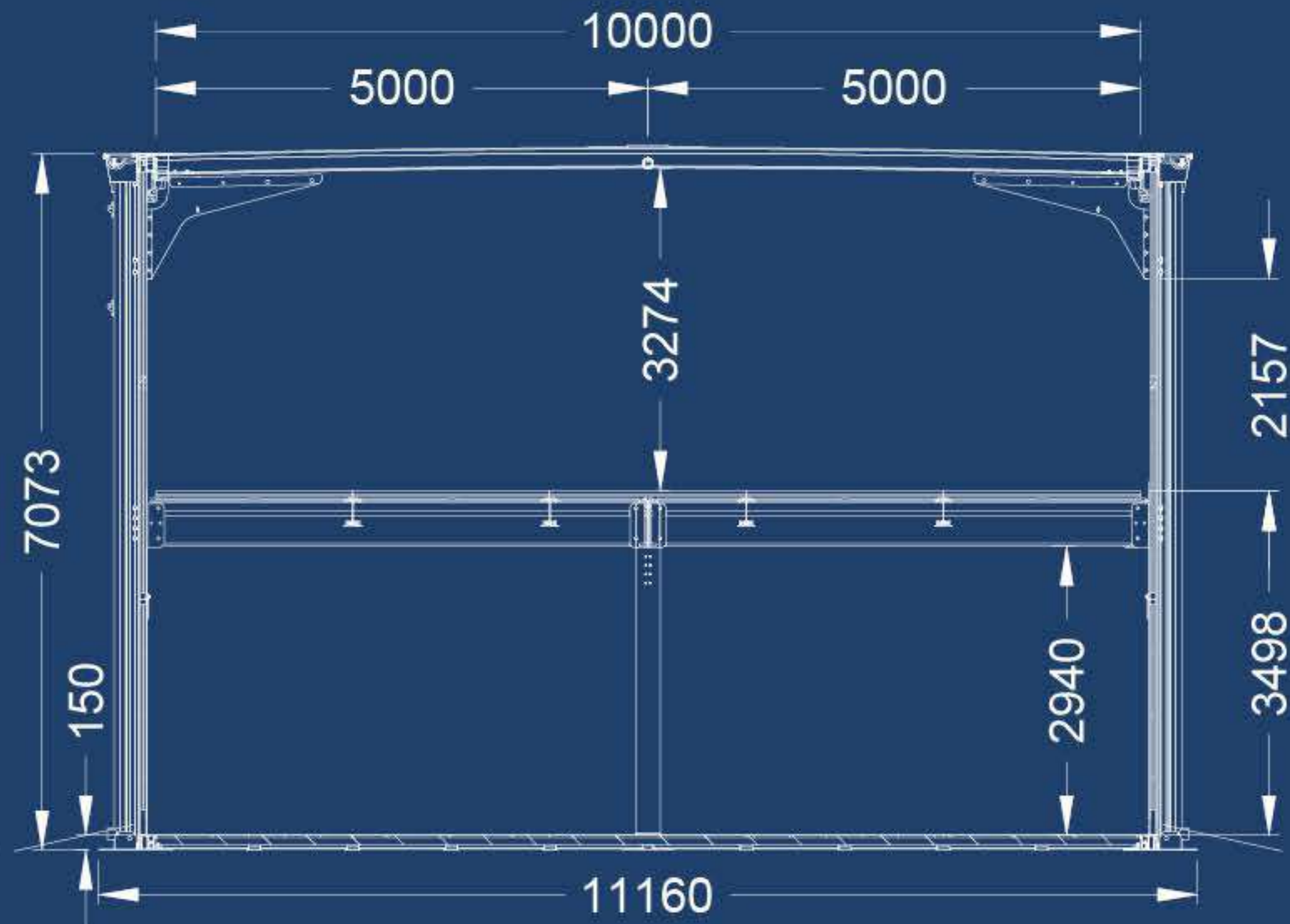
Pórtico de 10m con mezzanina
